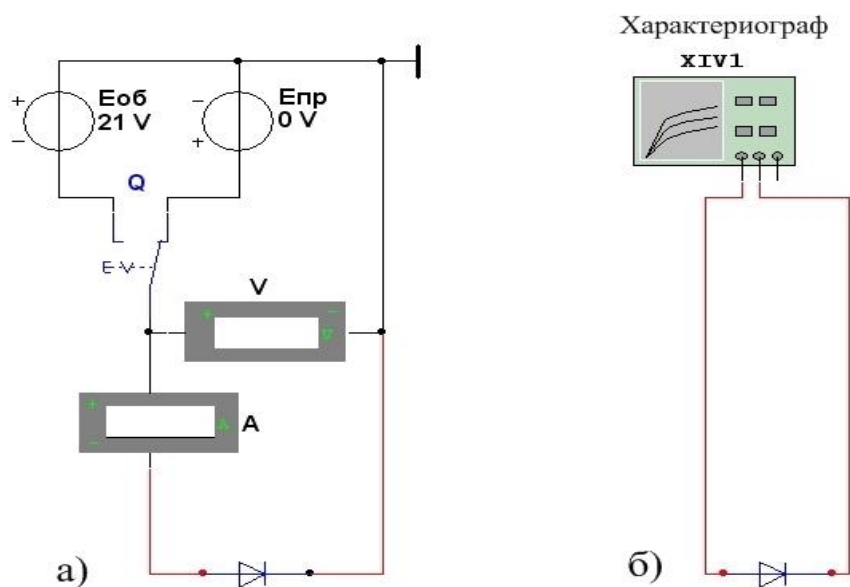
Рис. 6.2. Построение ВАХ диода: а) схема измерения, б) поиск интервала измерения с использованием характериографа
